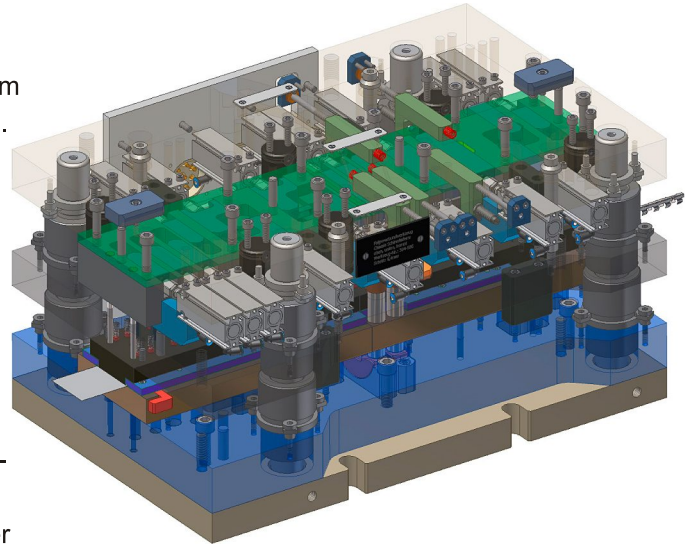
CAD-Zeichnung eines typischen Folgeverbundwerkzeugs aus dem Werkzeugbau von Rohde & Schwarz.
