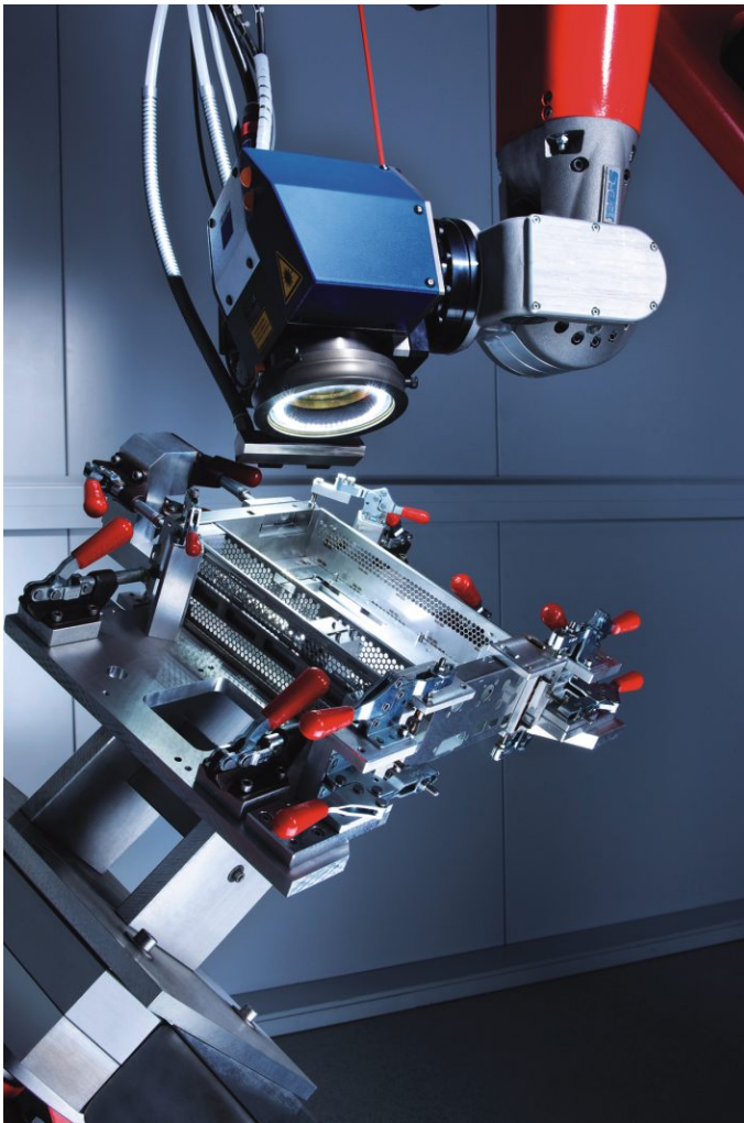
Laserschweißen mit Schweißvorrichtung (Alle Bilder: Rohde & Schwarz)
